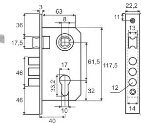
Basara 1023 M60Z NI (никель)
